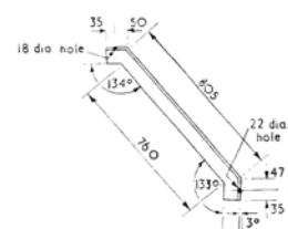
ITEM 11-60 x 60 x 8 Angle.
