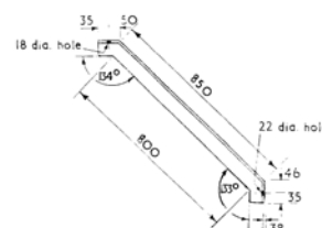
ITEM 9 - 60 x 60 x 8 Angle.
