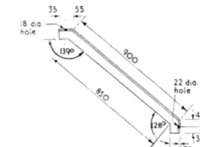
ITEM 7 - 60 x 60 x 8 Angle.
