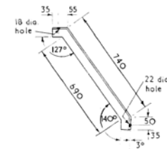
ITEM 12 - 50 x 50 x 8 ANGLE
